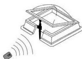
CLARABOYA DE APERTURA ELÉCTRICA CON MANDO A DISTANCIA
